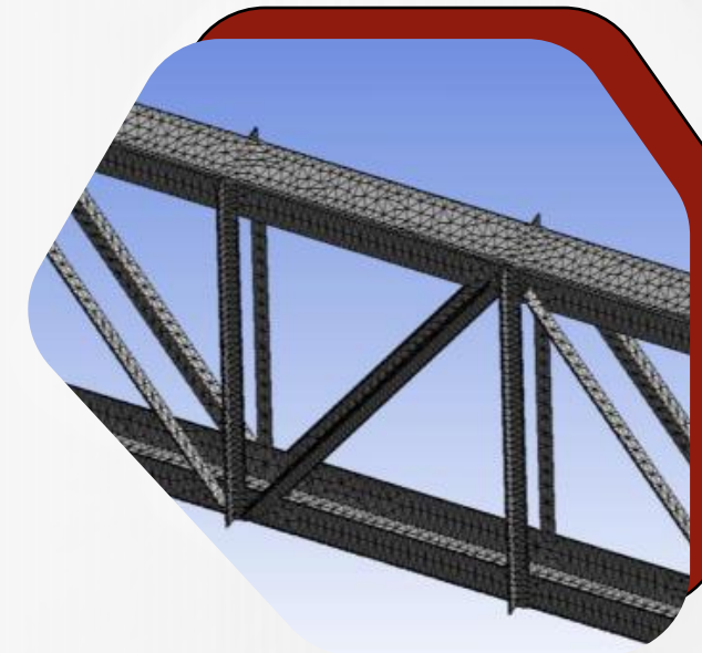
Modelagem e análise de estruturas por meio do método de elementos finitos
